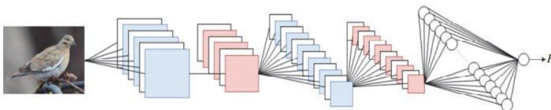
Рис. 1. Общая архитектура принципа работы сверточной нейронной сети
