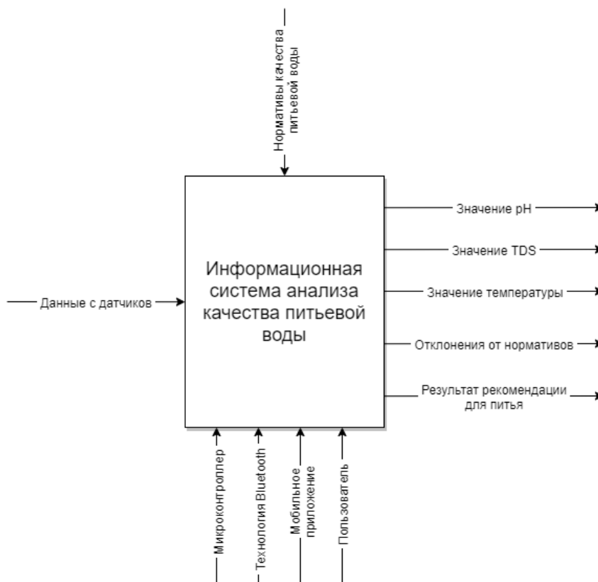
Рис. 1. Диаграмма IDEF0 ИС анализа качества питьевой воды.
