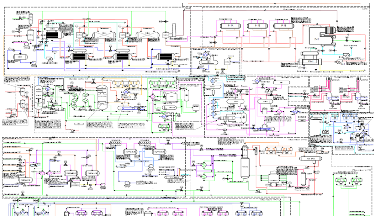
Рис. 1. Детальная модель части производства
