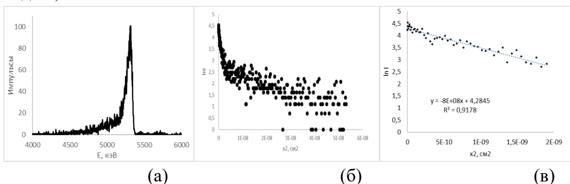
Рис. 1. Альфа-спектр сорбента MnO_2 -ТАЦ после сорбции Po -210 в кислой среде (а) и последовательная обработка и линейаризация (б, в)
