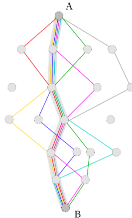
Рис. 5. Муравьиный алгоритм
