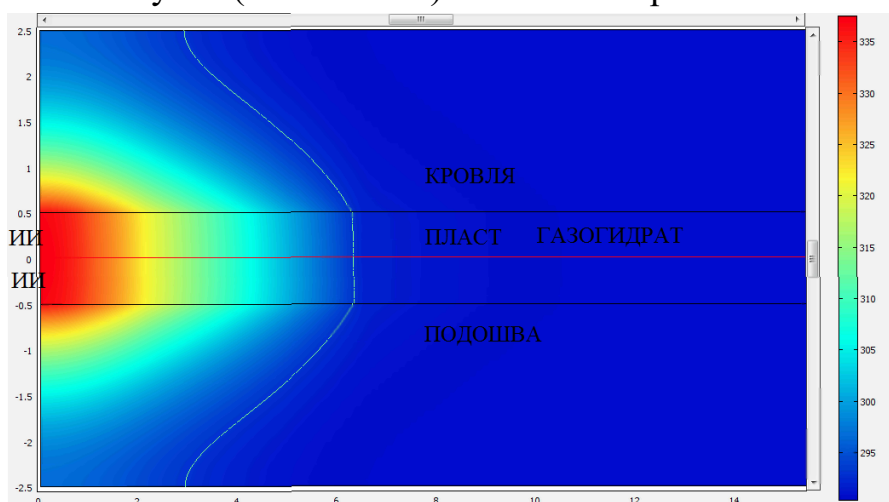
Рис. 1. Пространственное распределение температуры в газогидратном пласте в результате его нагрева источником электромагнитного излучения
